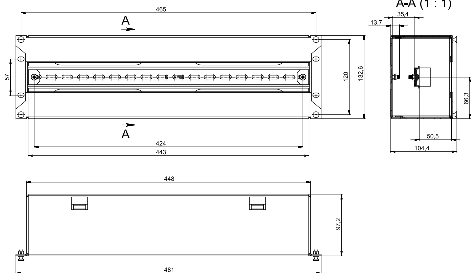
Технический эскиз
